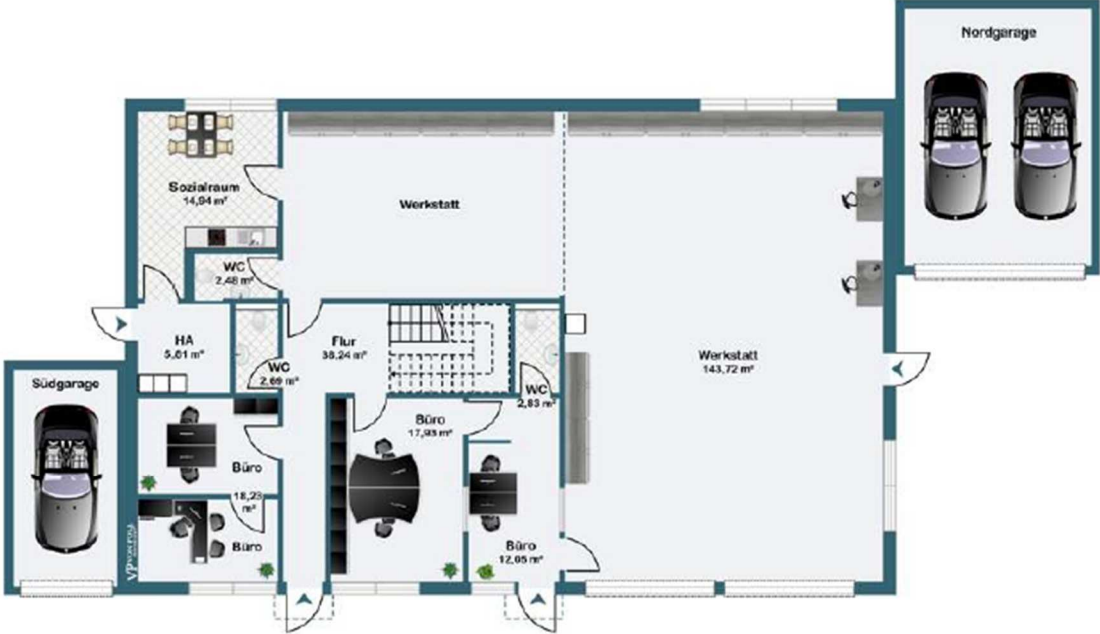
Erdgeschoss
