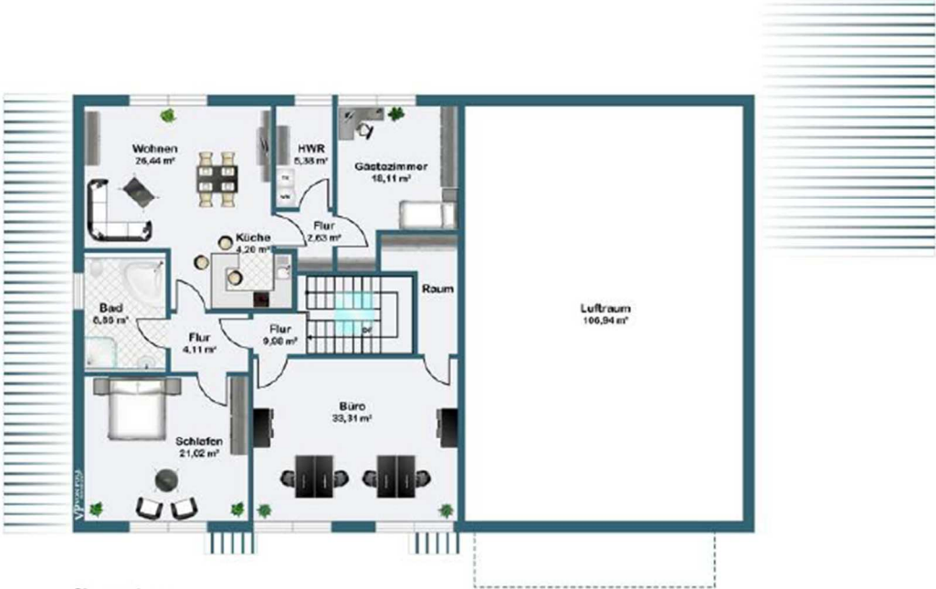
Obergeschoss
